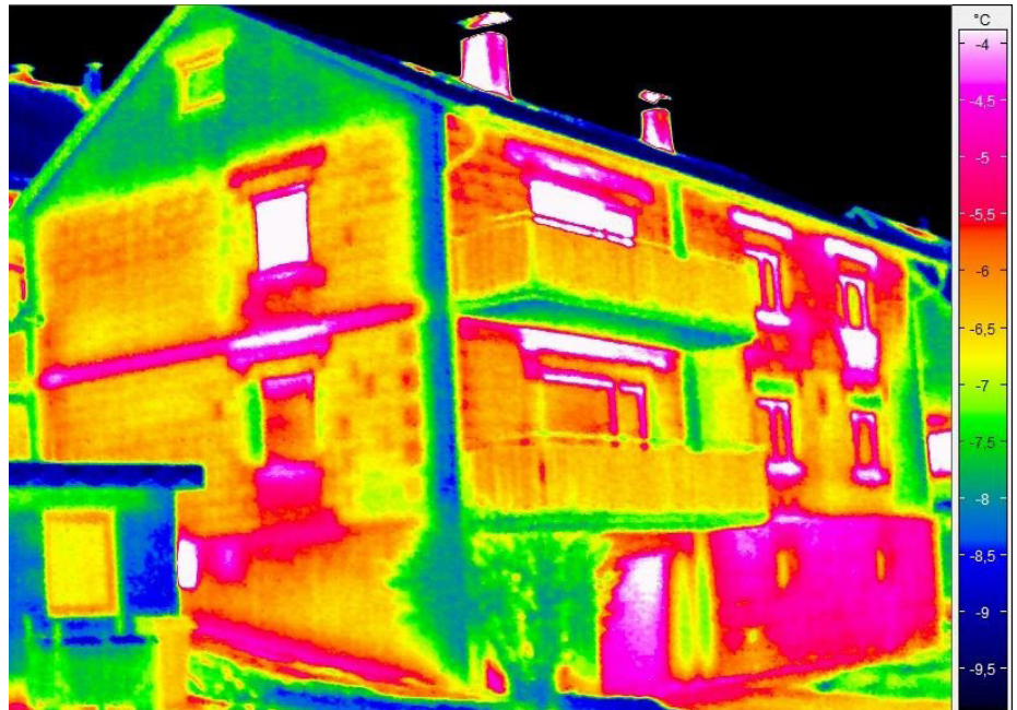
Thermografie eines Eschborner Hauses: Wärmeverluste sind in Rot dargestellt.
